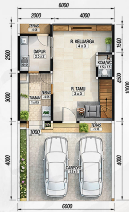
DENAH LT. 1 S 1 : 100
