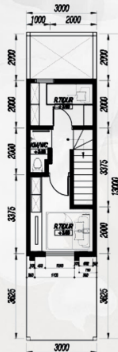
DENAH LT. 2 S 1 : 100
