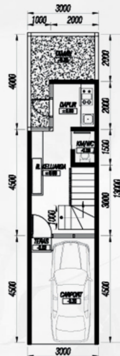
DENAH LT. 1 S 1 : 100
