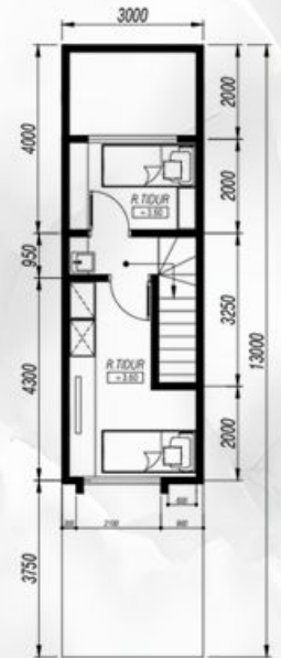
DENAH LT. 2 S 1 : 100
