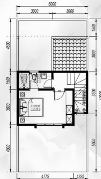
DENAH LT. 2 S 1 : 100
